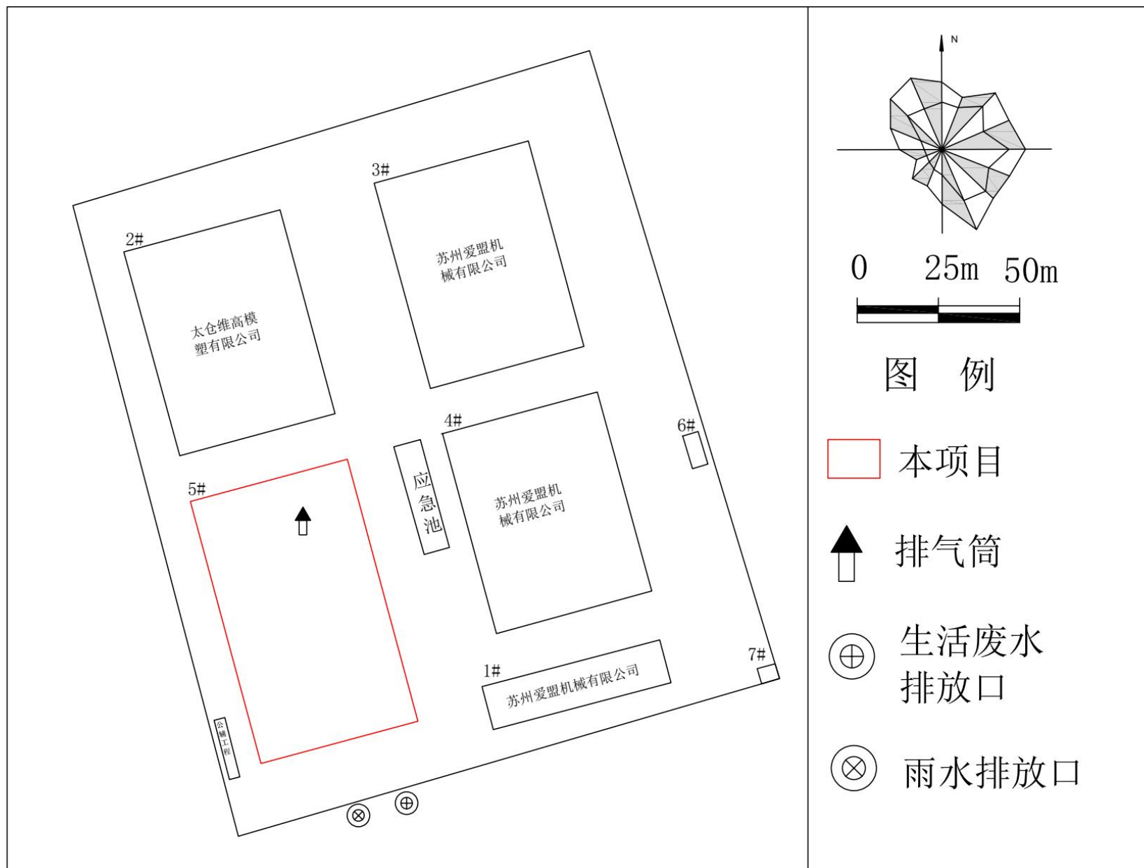
附图5 厂区总平面布置图
