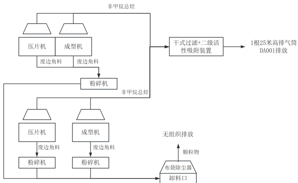
图 4-1 废气收集示意图
