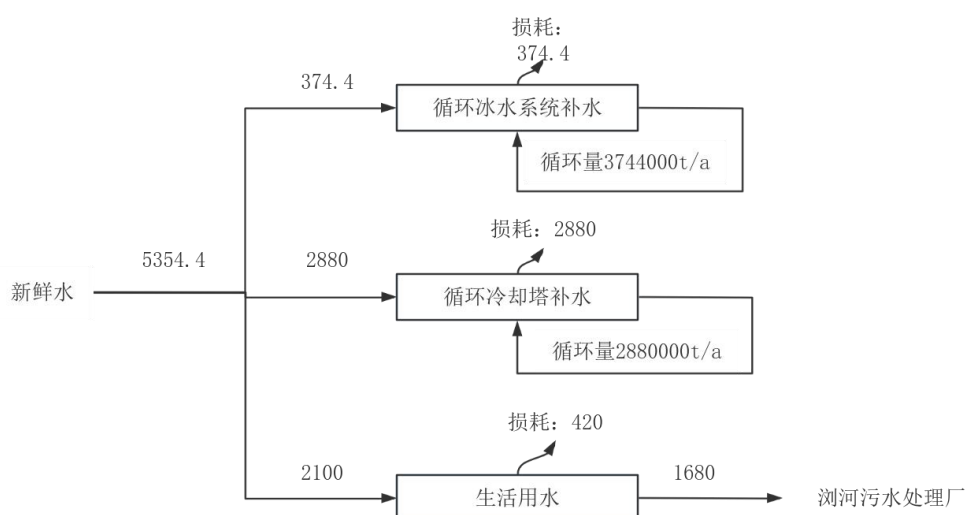
图 2-8 本项目水平衡图 (t/a)
