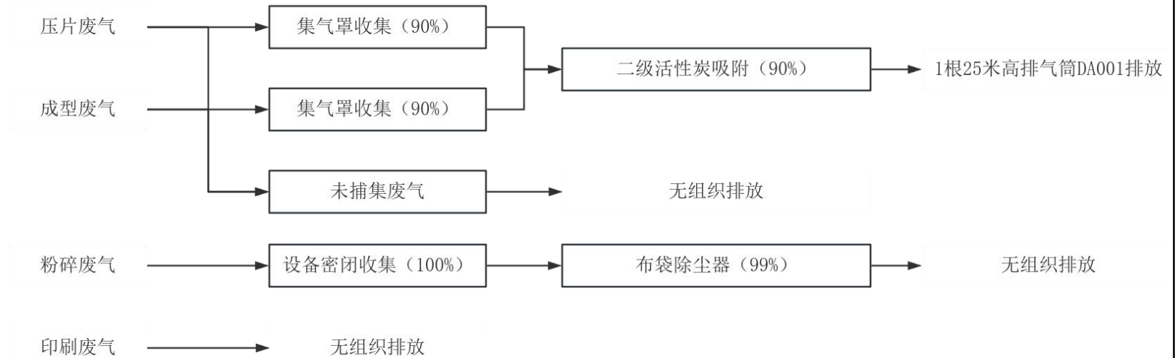
图 4-2 废气处理方式示意图
