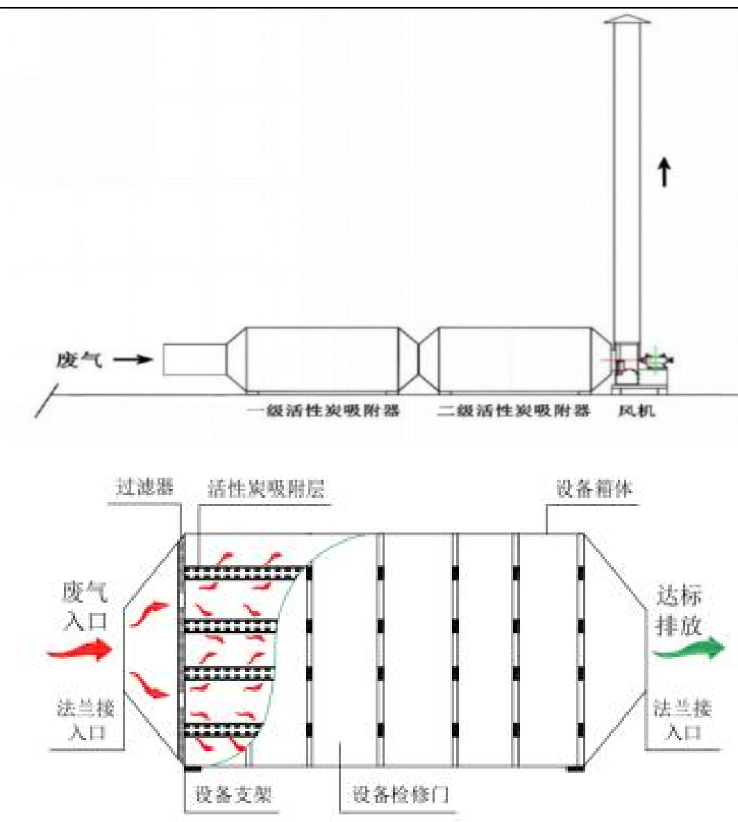
图 4-3 二级活性炭吸附工艺原理图
